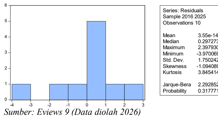
Hasil Uji Normalitas
